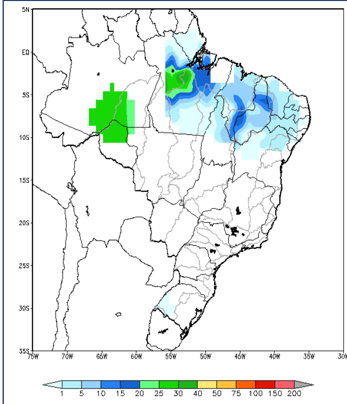
PRECIPITAÇÃO ACUMULADA (MM) OBSERVADA 28/01/2024
