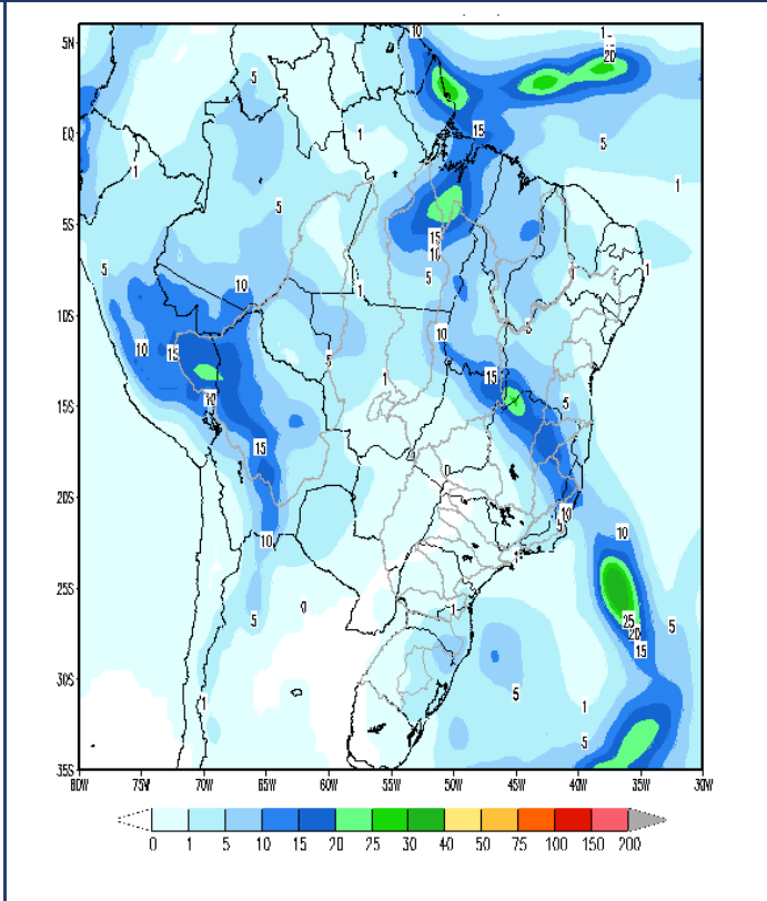
PRECIPITAÇÃO ACUMULADA (MM) PREVISTA 28/01/2024
