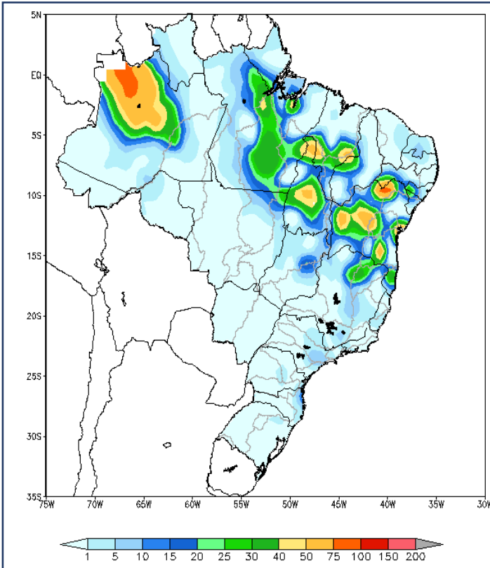
PRECIPITAÇÃO ACUMULADA OBSERVADA 20/01/2024 - 28/01/2024
