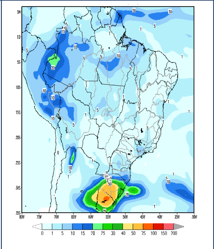
PRECIPITAÇÃO ACUMULADA (MM) PREVISTA 16/01/2024
