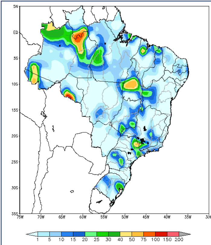
PRECIPITAÇÃO ACUMULADA OBSERVADA 13/01/2024 - 16/01/2024
