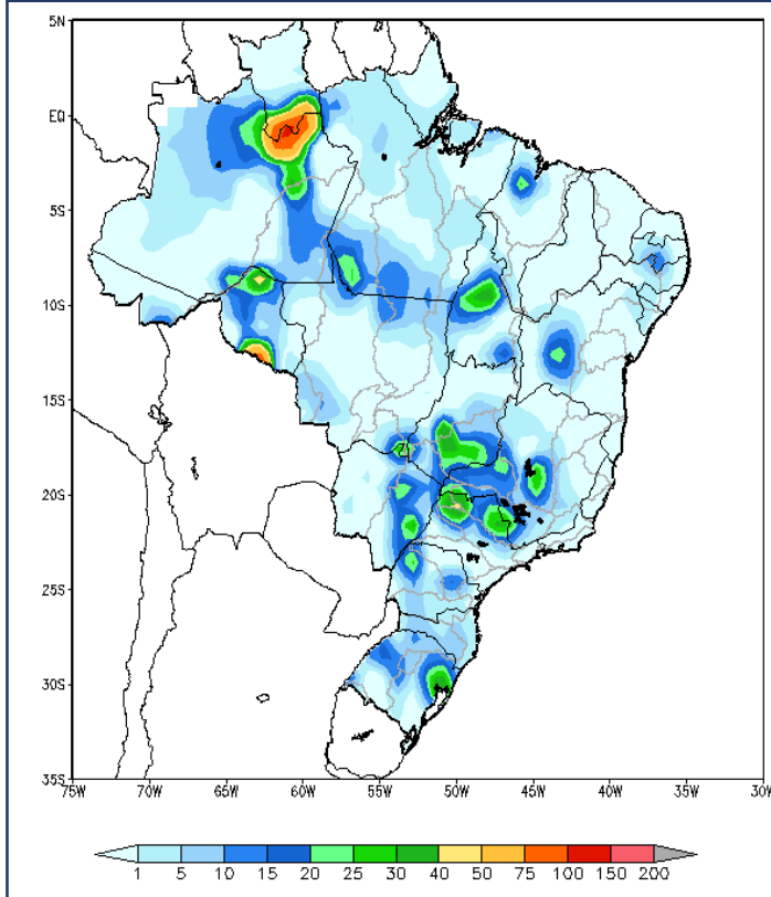
PRECIPITAÇÃO ACUMULADA (MM) OBSERVADA 16/01/2024
