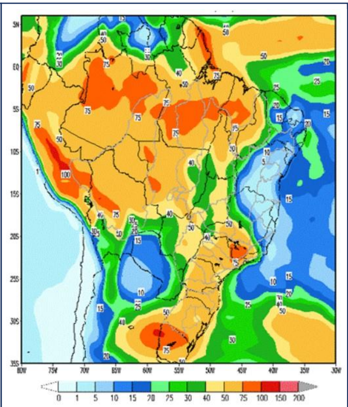
PRECIPITAÇÃO ACUMULADA PREVISTA 13/01/2024 - 19/01/2024
