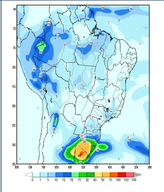
PRECIPITAÇÃO ACUMULADA (MM) PREVISTA 15/01/2024
