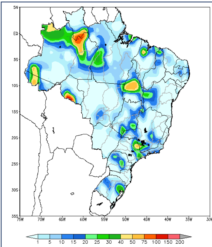
PRECIPITAÇÃO ACUMULADA OBSERVADA 13/01/2024 - 15/01/2024
